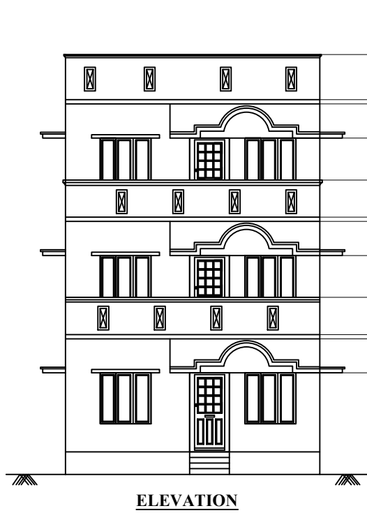
ELEVATION
