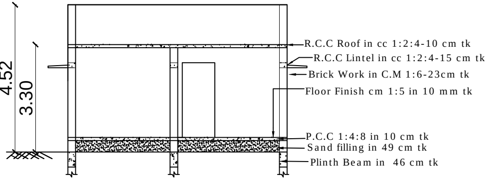
SECTION - AB
