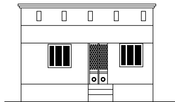
ELEVATION
