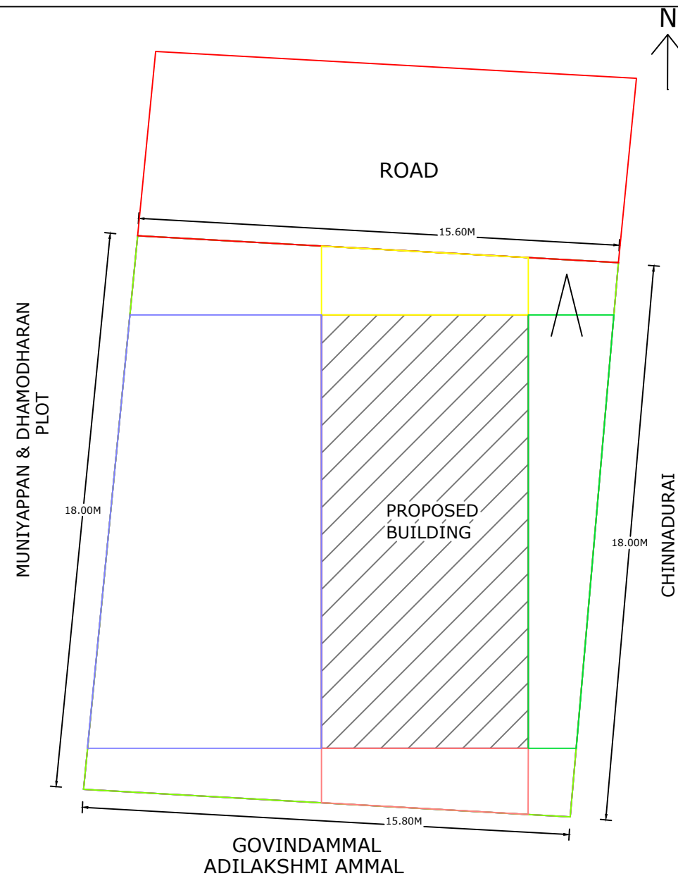
SITE PLAN: 1:100
