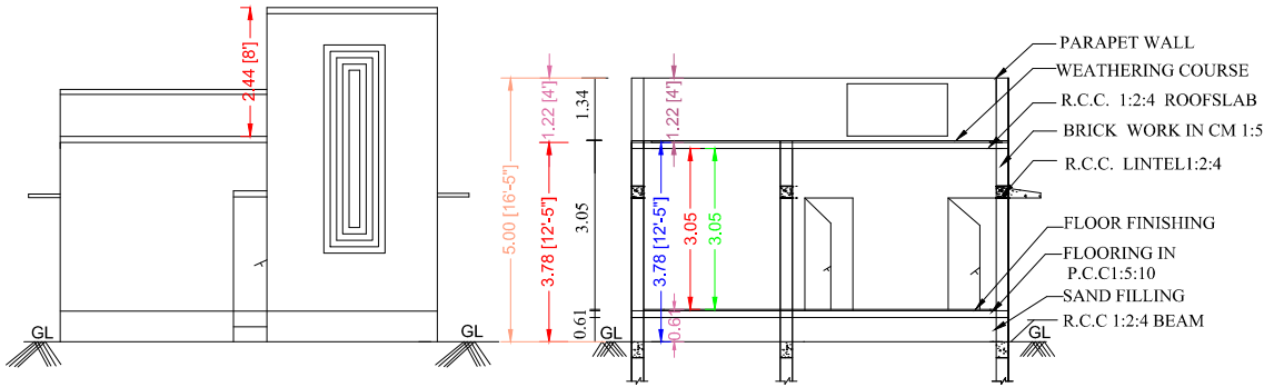
ELEVATION
