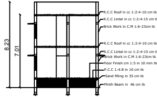
SECTION - AB
