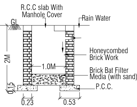
SCALE:- 1" = 4'0"
