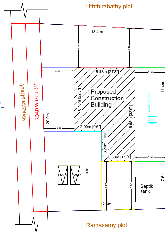
SITE PLAN:
