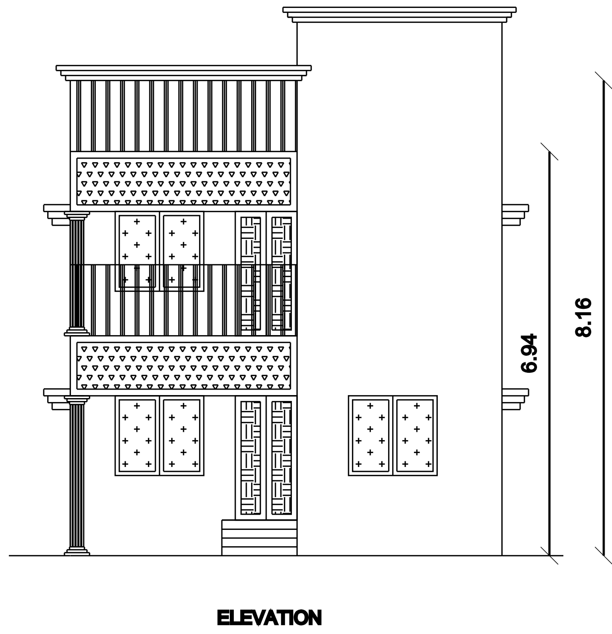
ELEVATION
