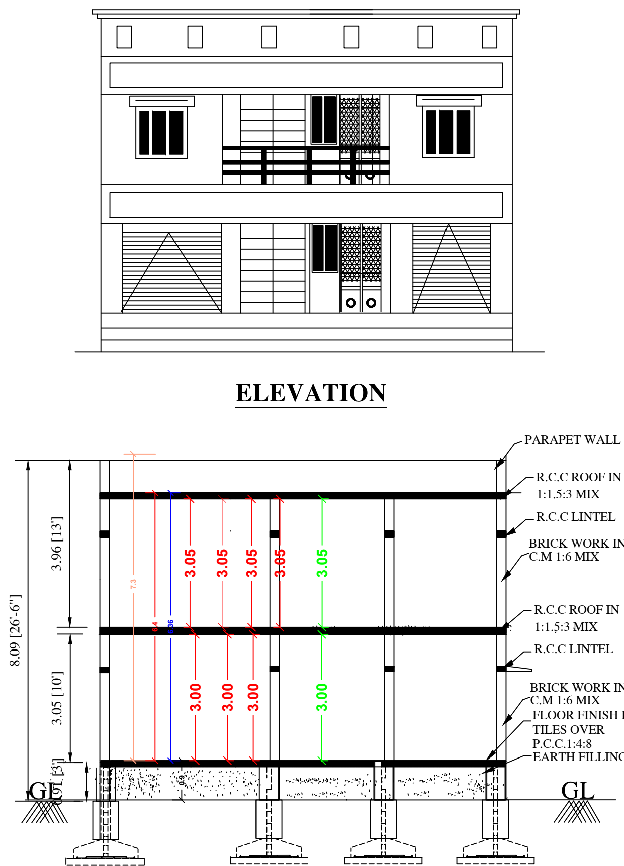
ELEVATION
