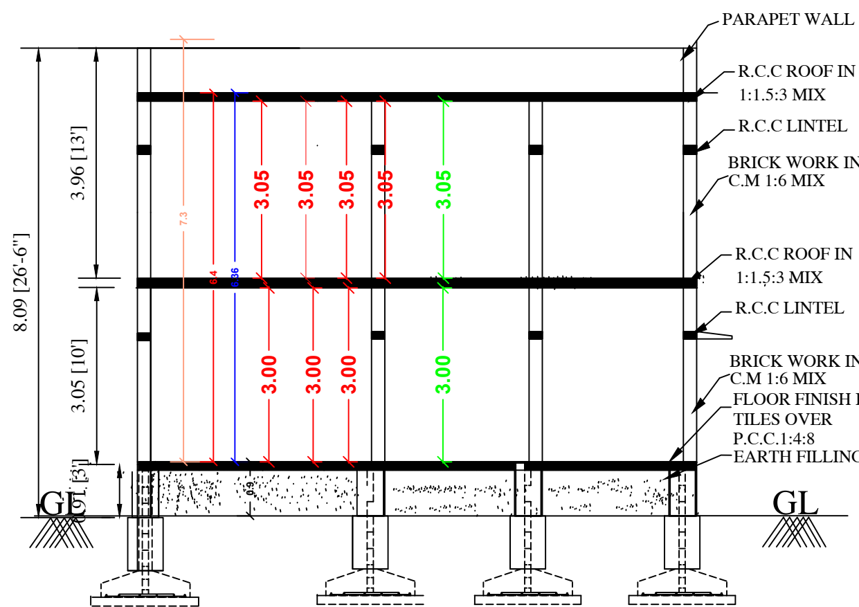
ELEVATION
