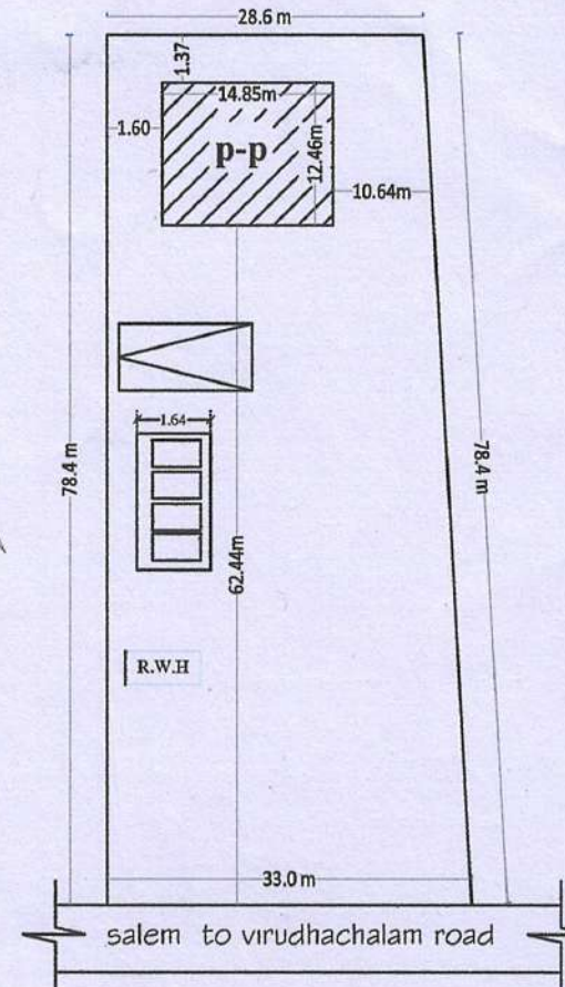
SITE- PLAN (N.T.S)
