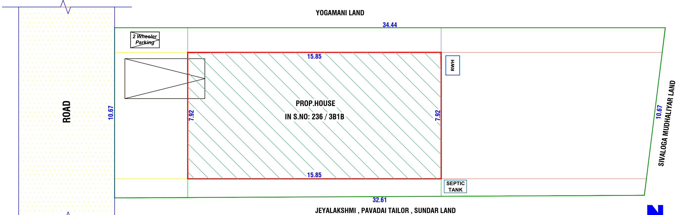
SITE PLAN SCALE 1:100
