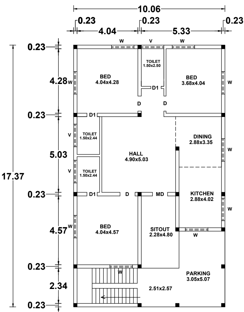
UND FLOOR PLAN
