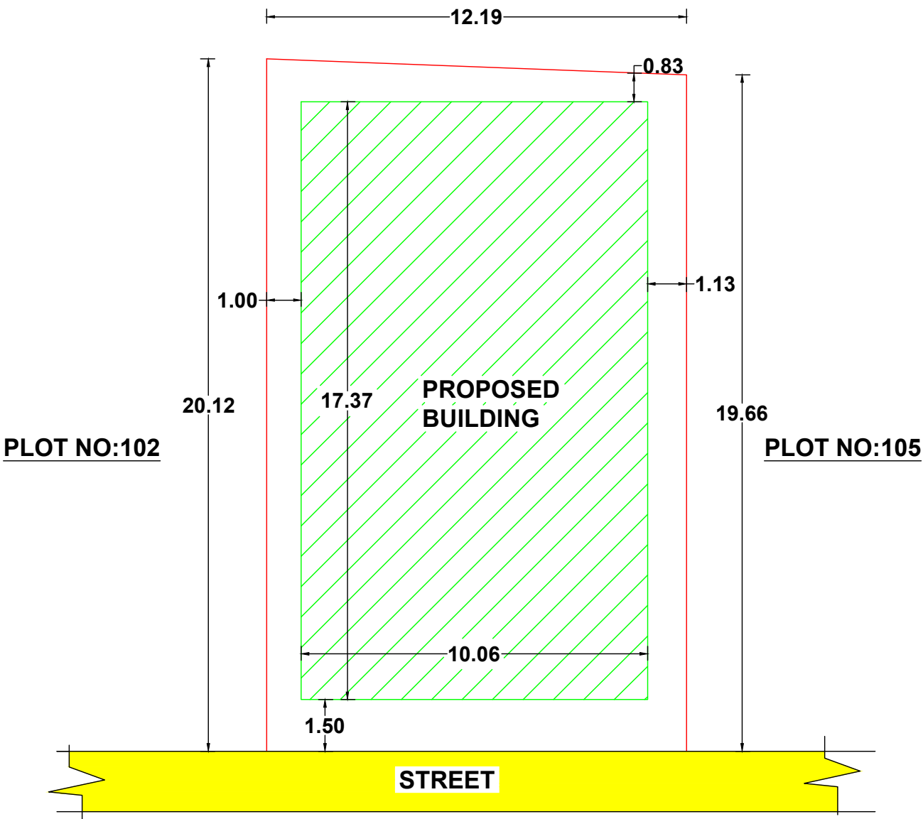
SITE PLAN 1:100
