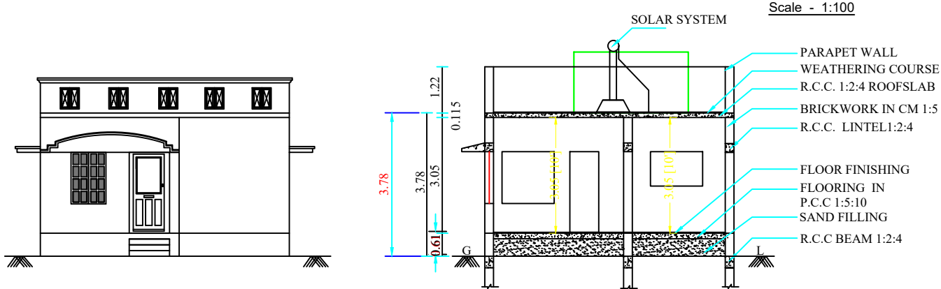
ELEVATION
