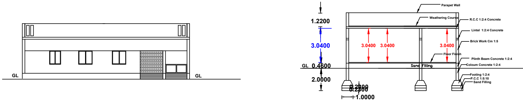
Elevation
