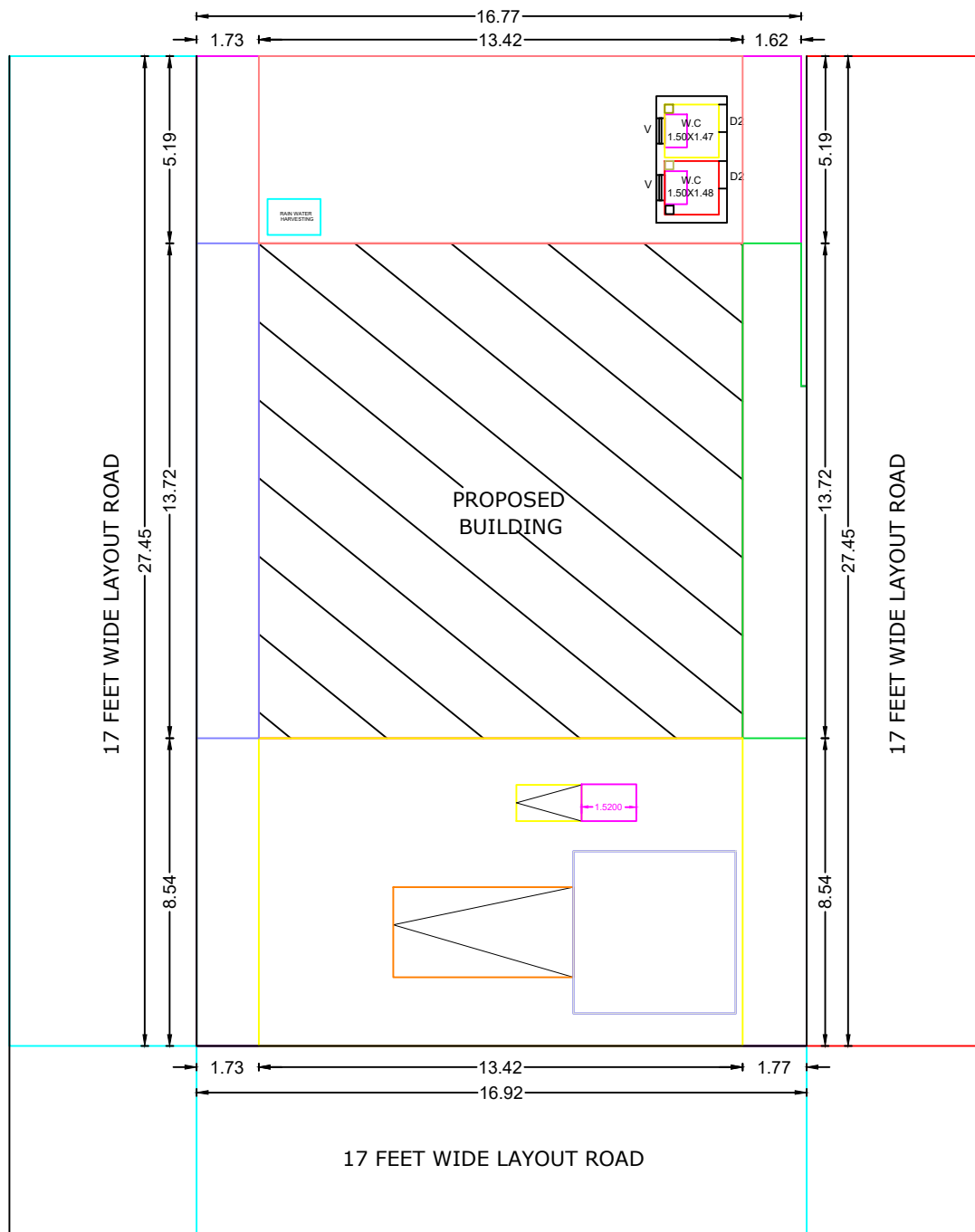
SITE PLAN:1:100
