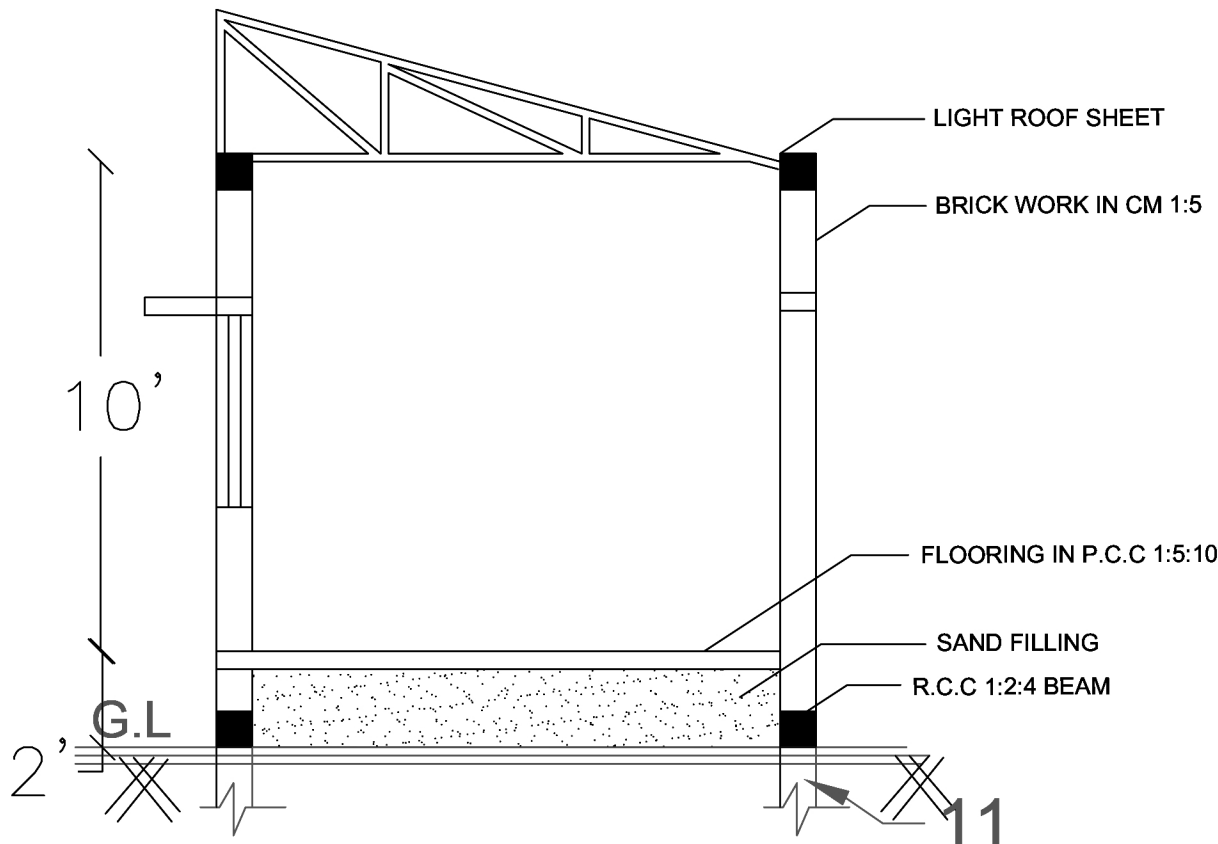
SECTION - AB
