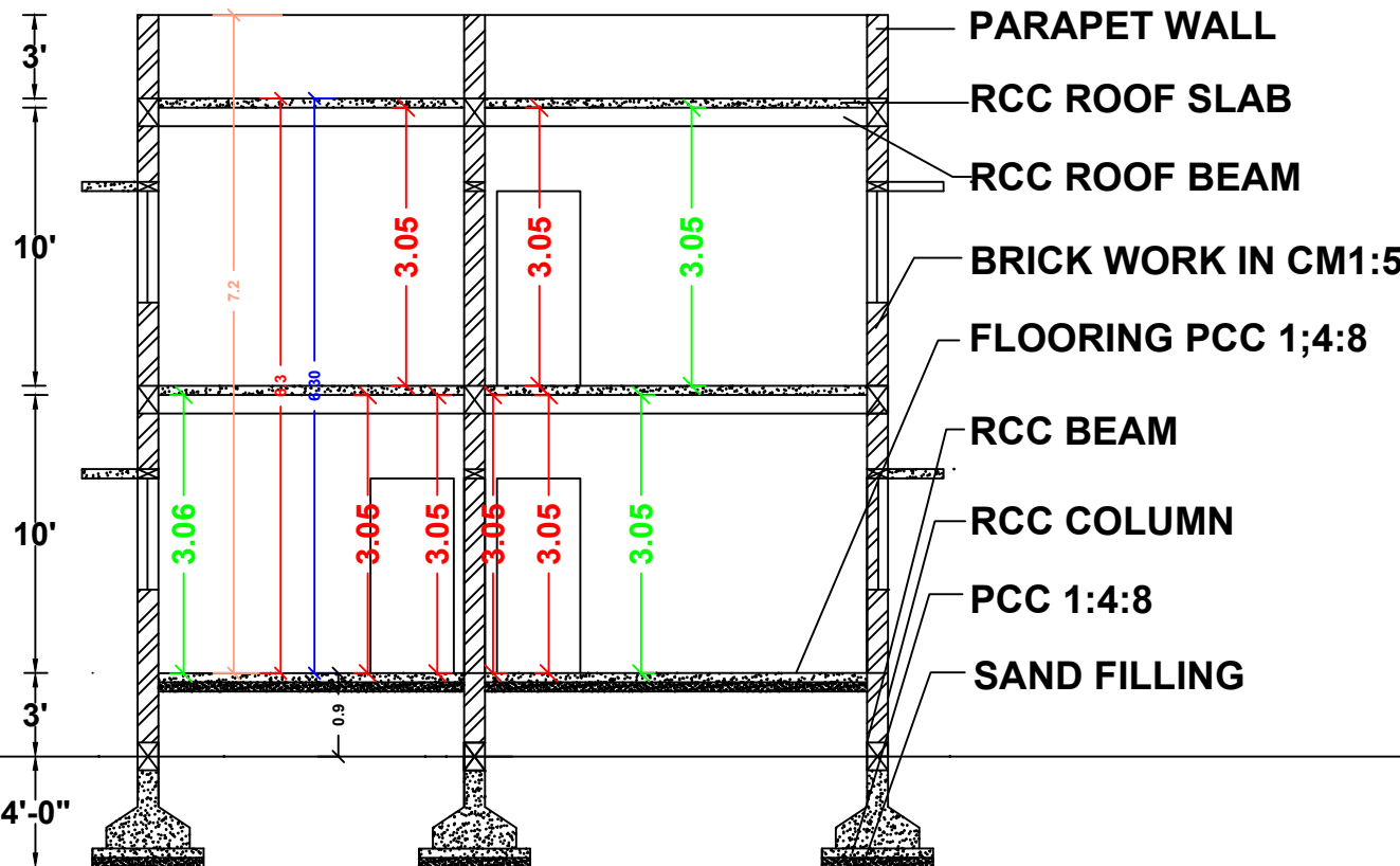
SECTION A-A
