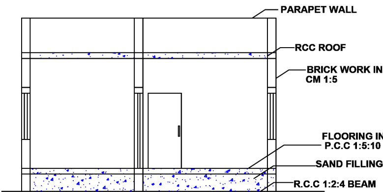
SECTION - AB
