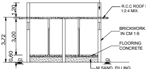
SECTION ON DD
