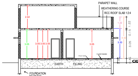
SECTION A-B
