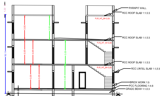
SECTION A-A' B-B' C-C'
