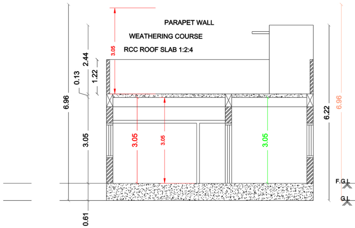
SECTION ON-'A'B'
