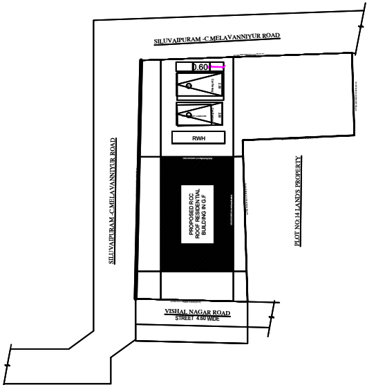
SITE PLAN.
