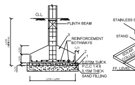
TYP. DET. COLUMN FOOTING
