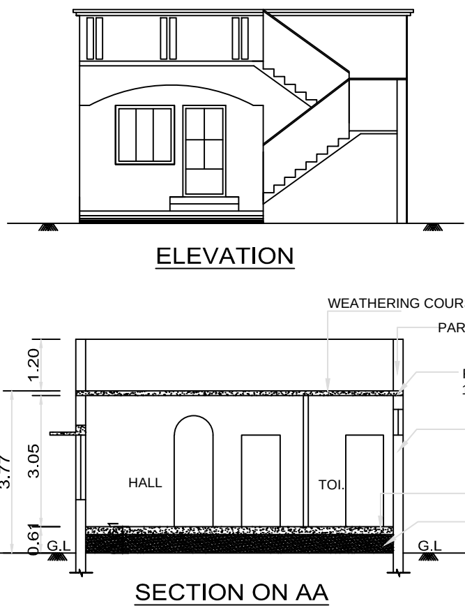
ELEVATION
