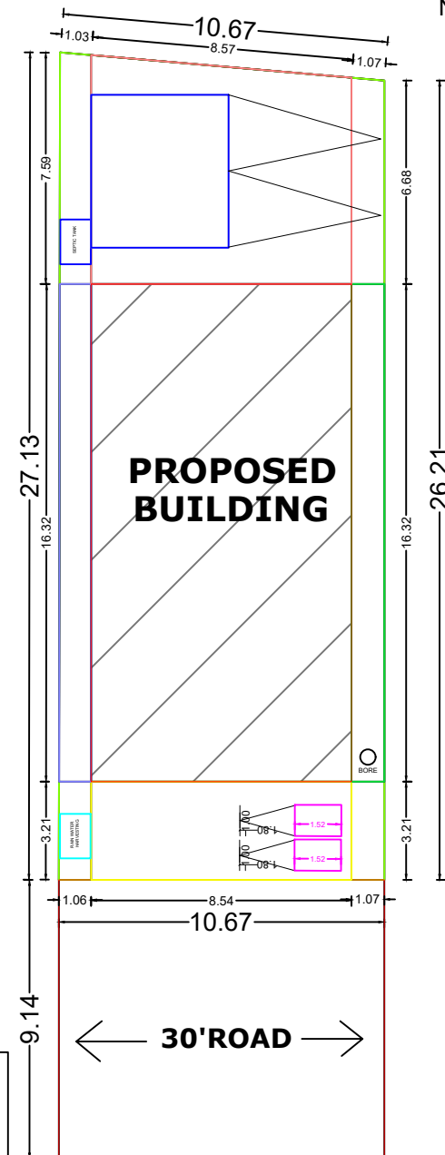
SITE PLAN: 1:100
