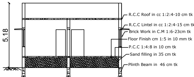
SECTION - AB
