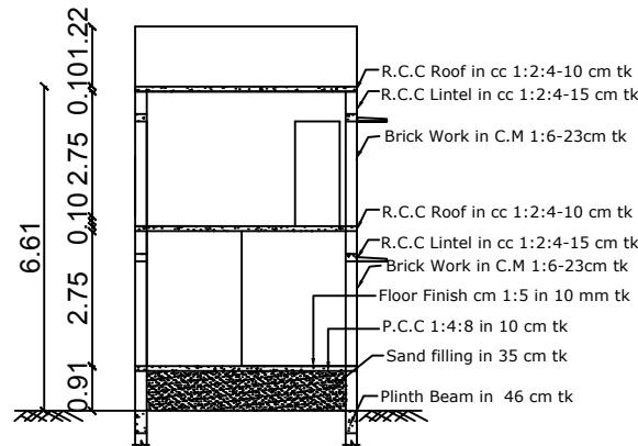
SECTION - AB
