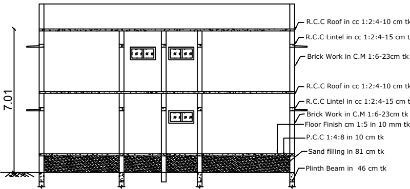
SECTION - AB
