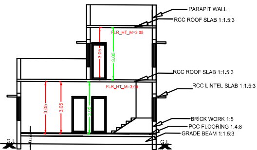
SECTION A-A' B-B'
