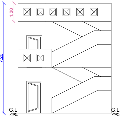
ELEVATION
