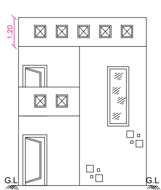
ELEVATION
