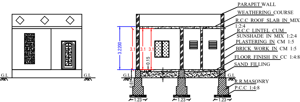
SECTION - AB
