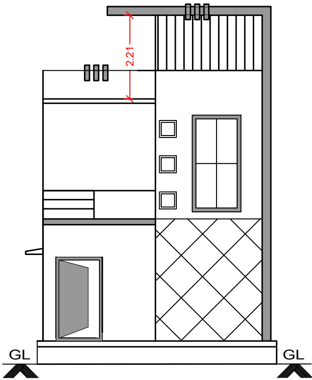
ELEVATION-A
