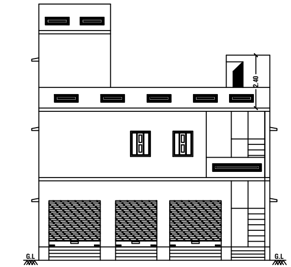
ELEVATION
