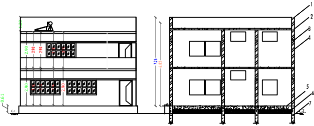
ELEVATION
