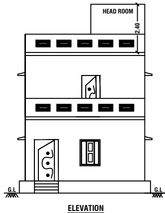
ELEVATION
