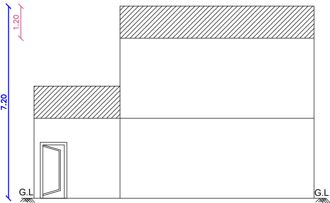
ELEVATION
