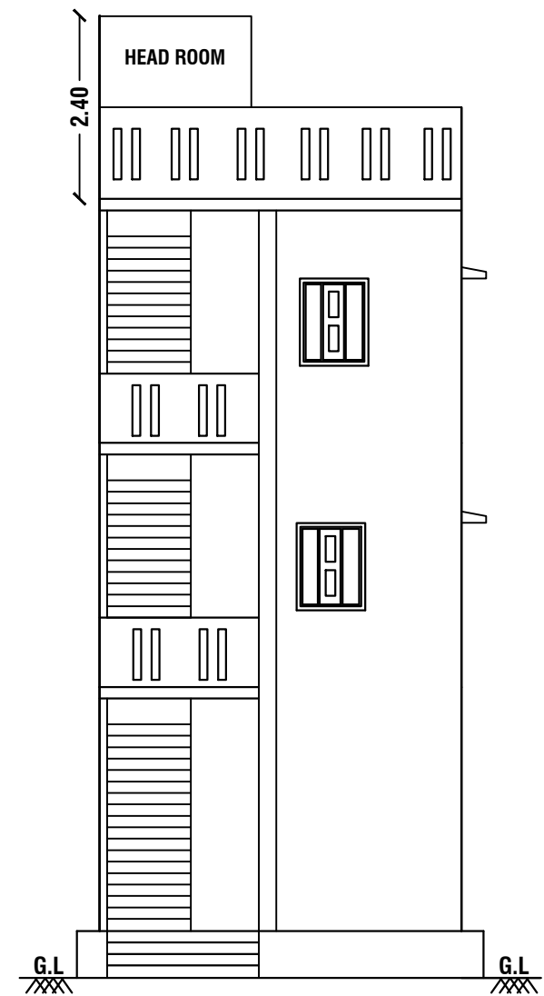
ELEVATION
