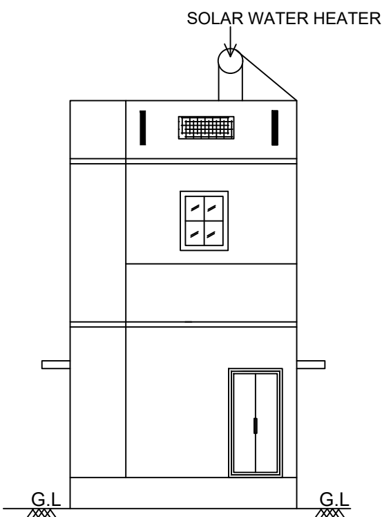
Elevation
