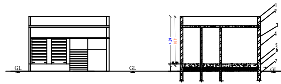
ELEVATION
