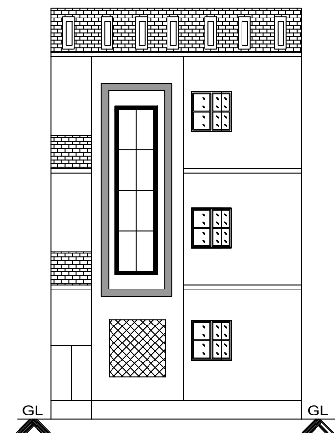
ELEVATION-A
