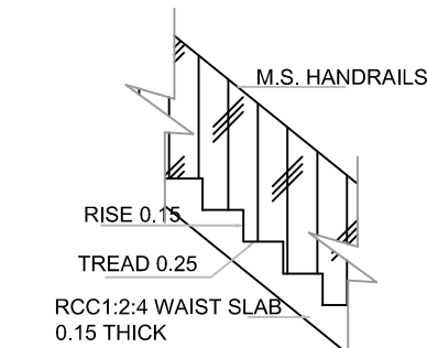
STAIRCASE DETAILS SCALE: 1:20
