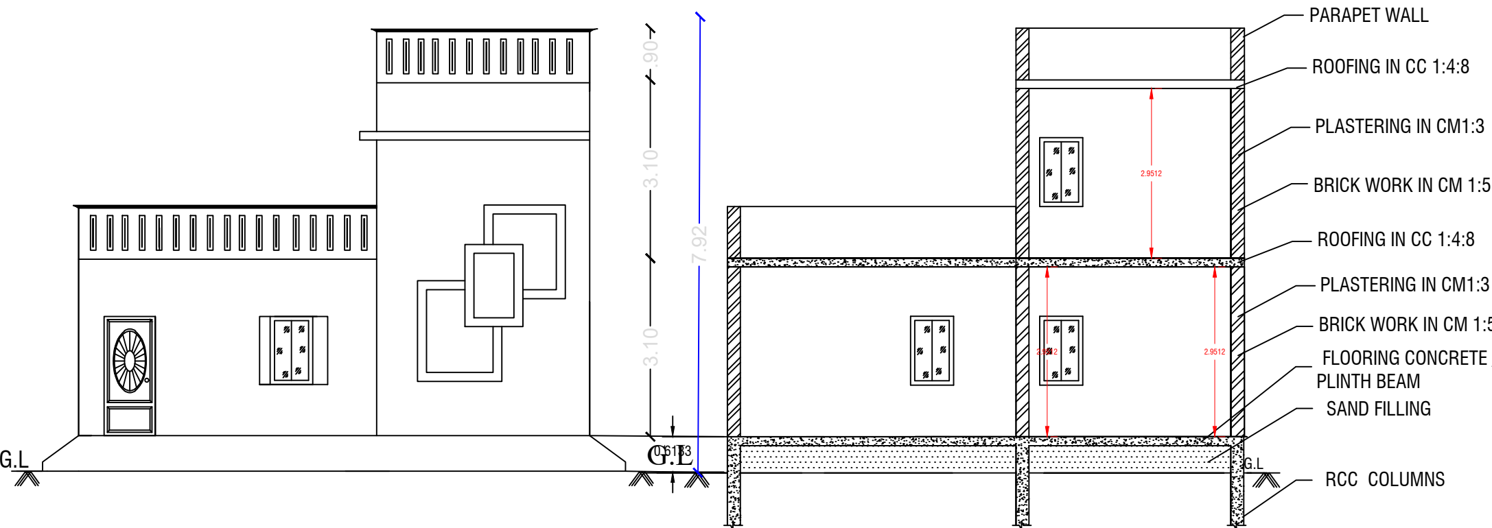
ELEVATION
