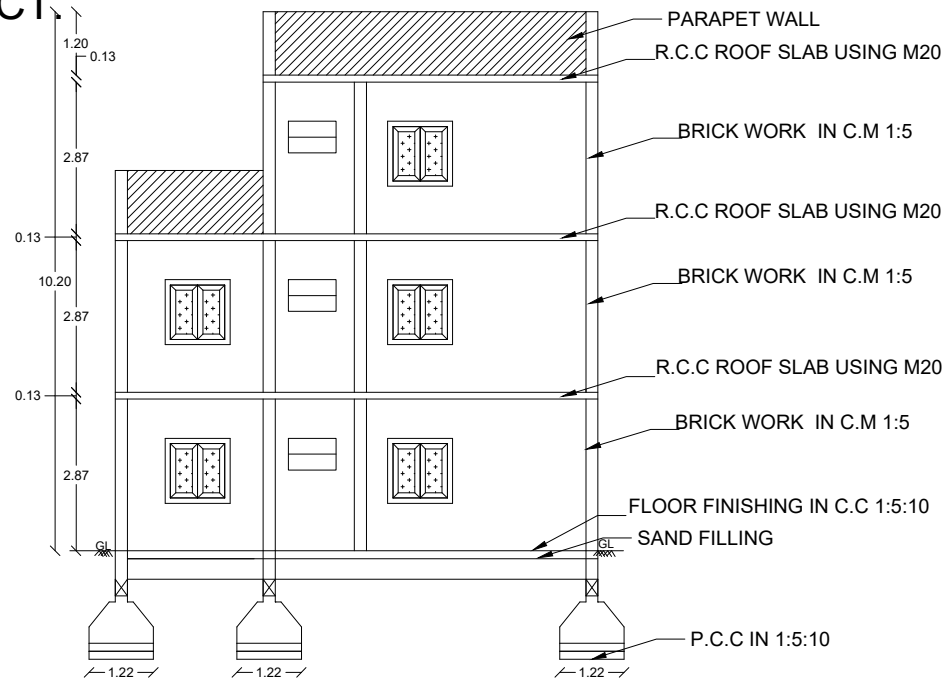
SECTION A-A
