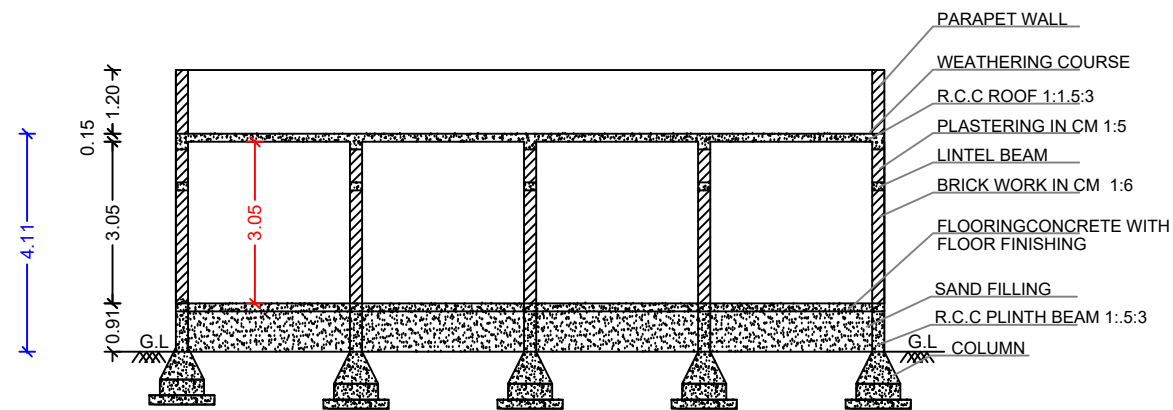
SECTION A-A'
