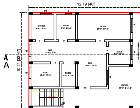
EXISTING G.F PLAN
