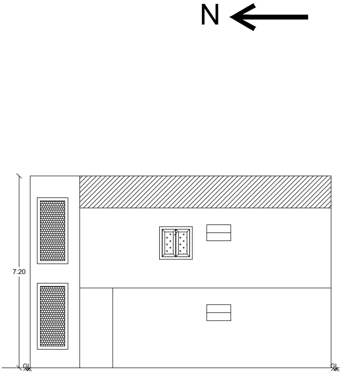
ELEVATION
