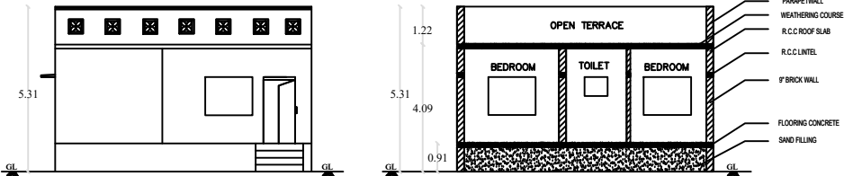
ELEVATION
